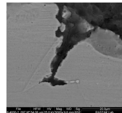
تصویر SEM-BSE در بزرگ نمایی ۵۰۰۰ برابر
